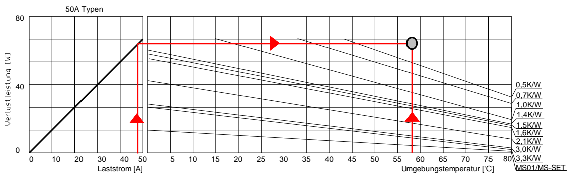
Abbildung 10 - Beispiel Kühlanforderung PR4850
