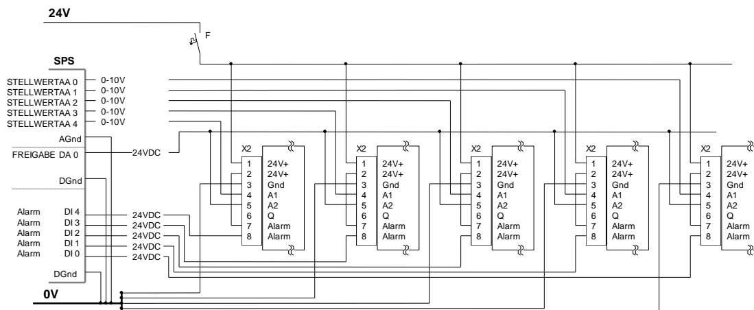
Abbildung 8 - Ausführung mit individueller Alarm-Auswertung
