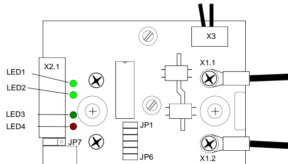
Abbildung 13 - Bedeutung der LEDs
