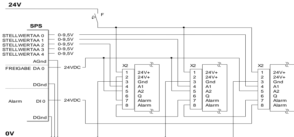
Abbildung 9 - Ausführung mit Summen-Alarm-Auswertung
