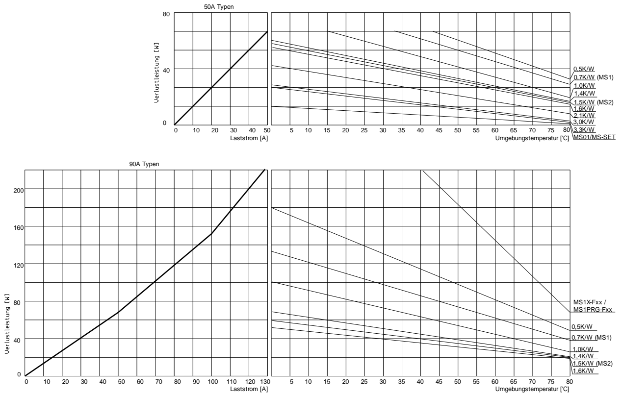
Abbildung 6 - Derating Kurven
