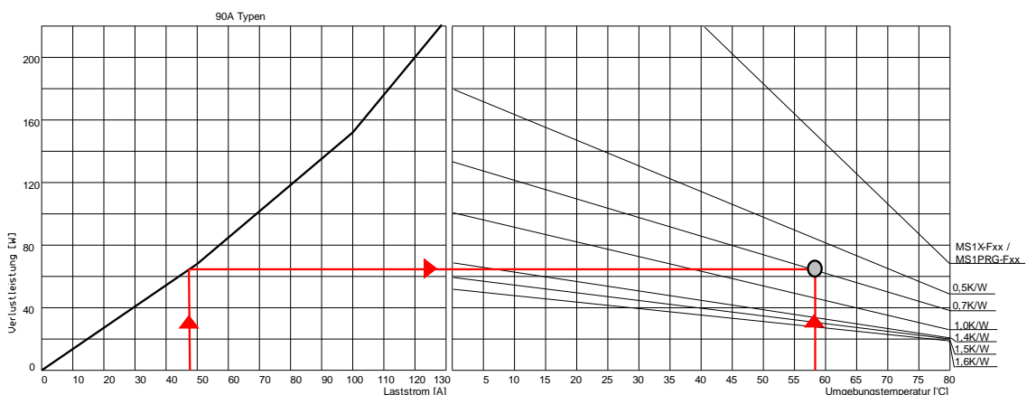
Abbildung 11 - Beispiel Kühlanforderung PR4890
