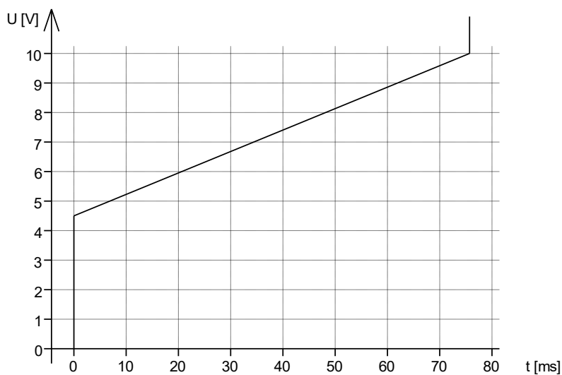
Abbildung 12 - Rampenzeit als Funktion der Steuerspannung
