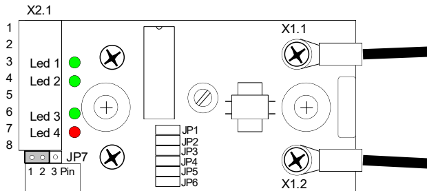
Abbildung 18 - Bedeutung der LEDs
