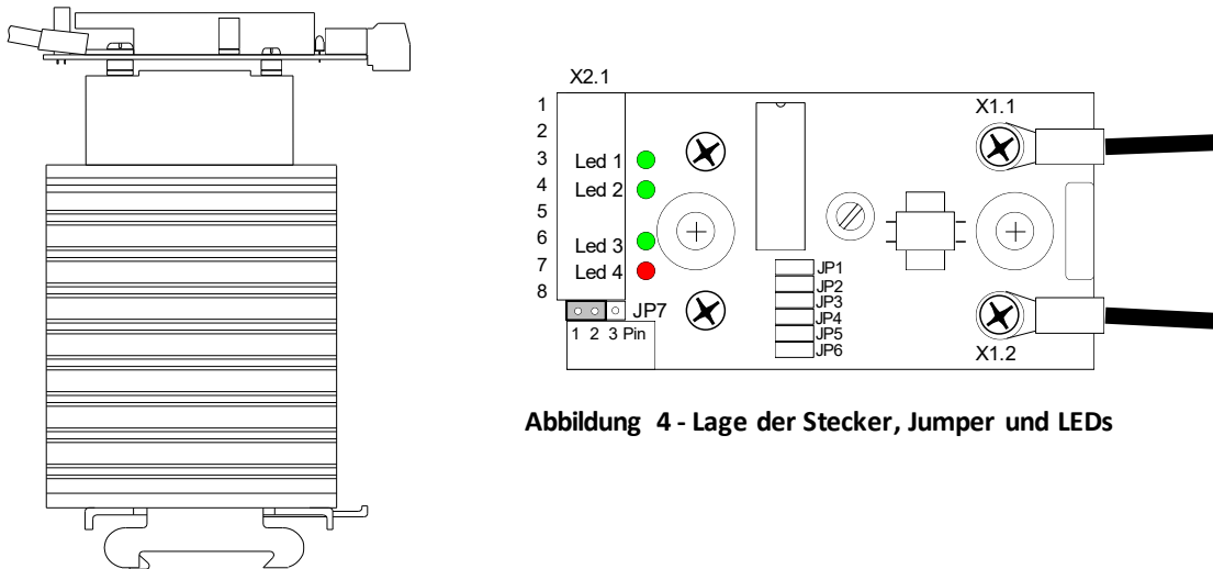
Abbildung 5 - Ausführungsbeispiel HP4075-3201
