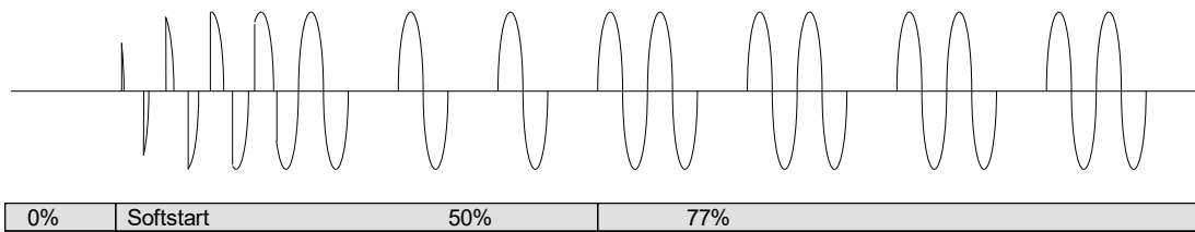
Abbildung 9 - Darstellung der Pulspaketsteuerung mit Sanftanlauf
