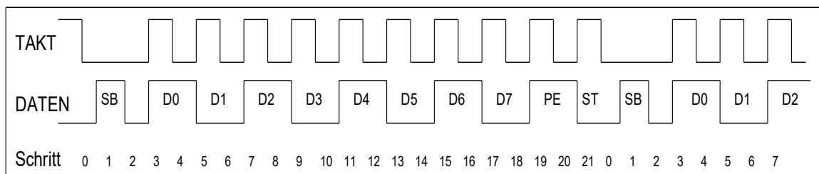
Abbildung 2 - Serieller Telegrammaufbau des TransDil-Protokolls
